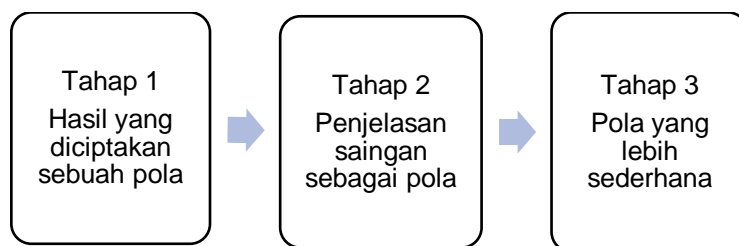
Gambar 2. Tahapan analisis data menggunakan Pattern Matching (Sumber:Yin, 2014)
